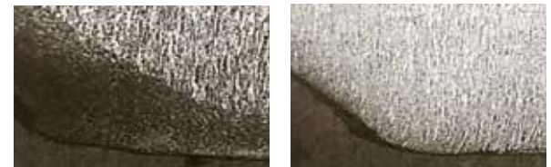
Cu-Cr-Zr nach 1200 Schweißungen
