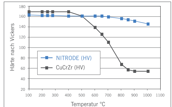
Härte bei hoher Temperatur
