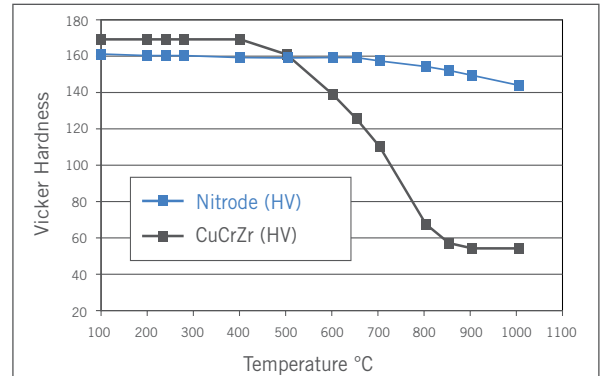
高温での硬度
